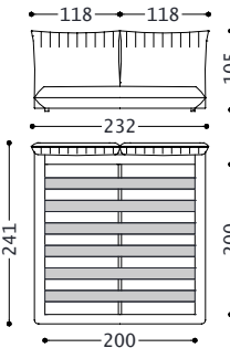
1BVLLA200A 2BVPLA200A
