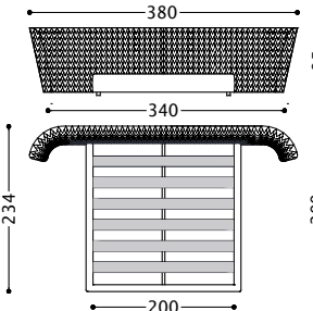
1SM2LA200
